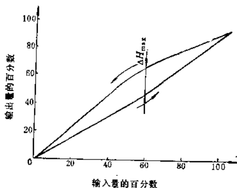
图1-3-3 迟滞误差
