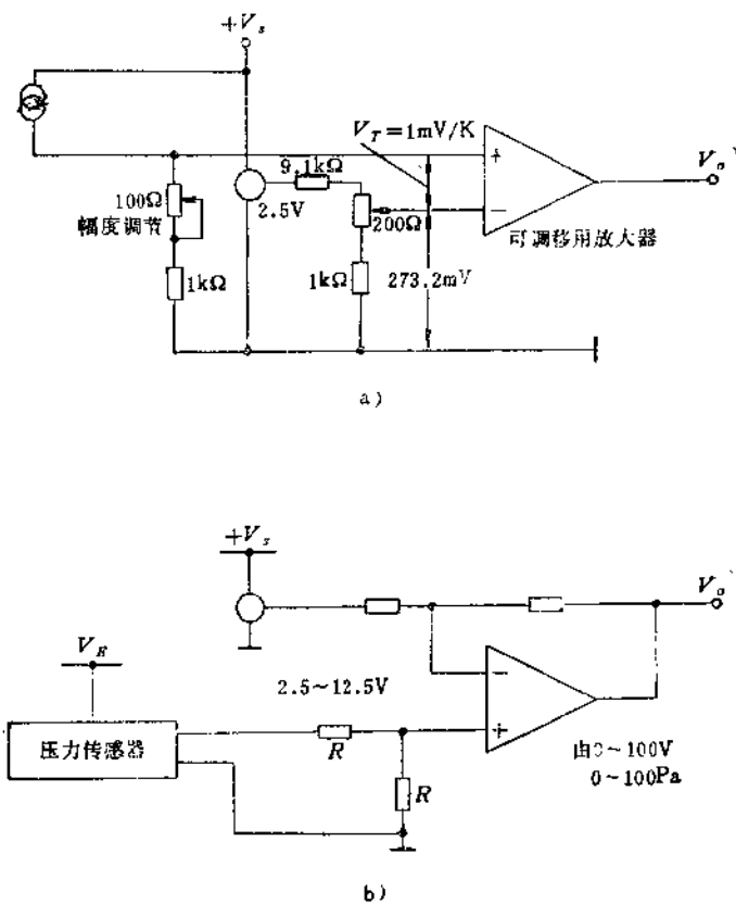
图1-3-68 量程偏置
