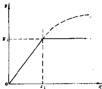
图 1-3-12 饱和特性
